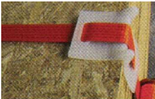
כיסוי פינות של המטען (המלצה) אמצעי כיסוי הפינות יהיו עשויים מעץ, מפלסטיק, ממתכת קלה (סגסוגת) או מחומר מתאים אחר לצורך מניעת שחיקה של התקן הריתום בחיכוך עם פינות חדות של המטען ובכך מניעת סיכון לחיתוך התקן הריתום או לנזק למטען.
